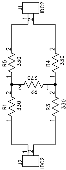
10 Db Attenuation
